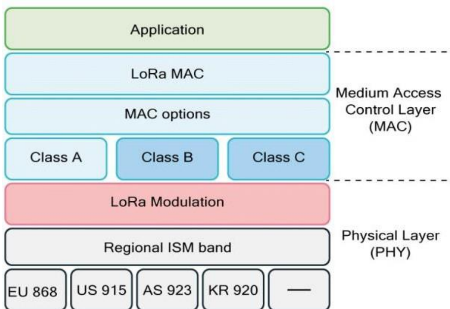
Slika 2. 2 LoRaWAN arhitektura[1]
