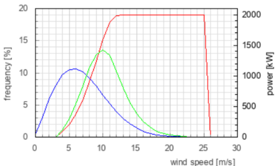
Slika 5.8.- Karakteristične krivulje snage i Weibullove funkcije za A= 8 m/s, k=2 [19]
