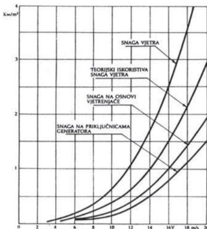
Slika 2.6.- Ovisnost snage vjetra o brzini [13]
