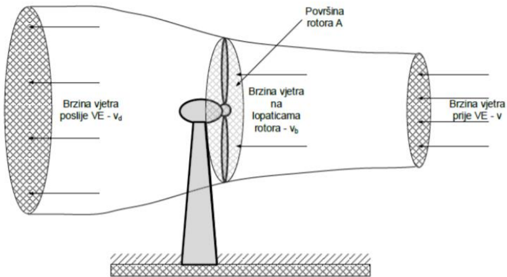
Slika 2.1.- Učinkovitost vjetroturbine [8]
