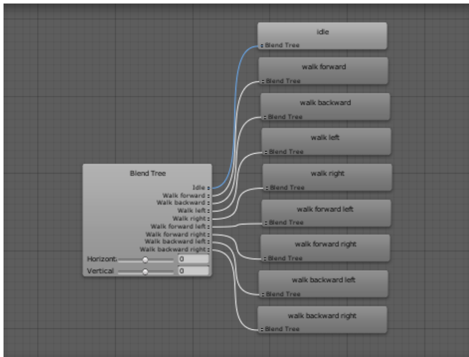
Slika 31: Nazivi animacija
