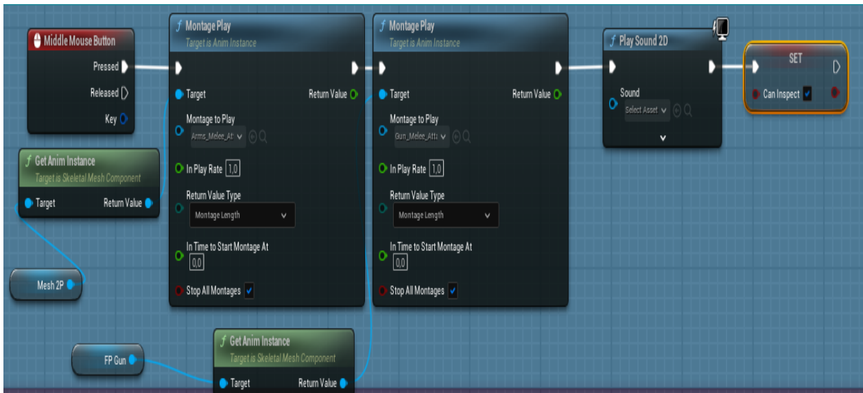
Slika 14: Implementacija mehanike bliskog napada
