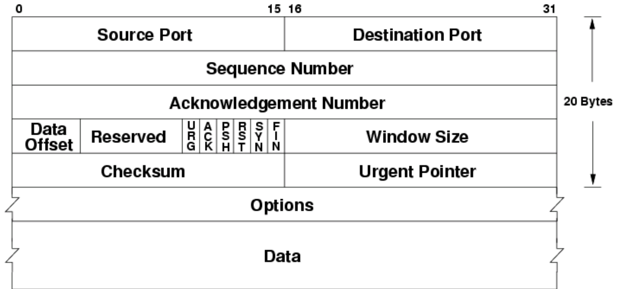
Slika 3.3. TCP protokol
