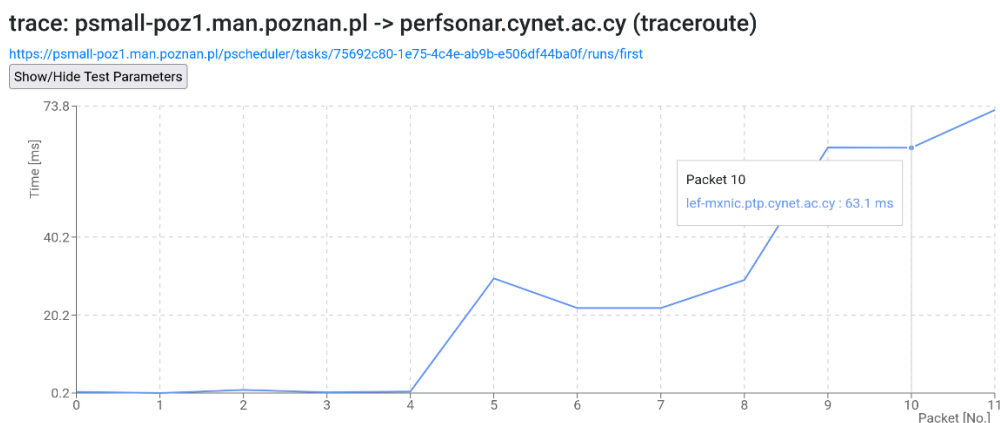
Slika 4.7. Mjerenje traceroute -a između Poljske i Cipra
