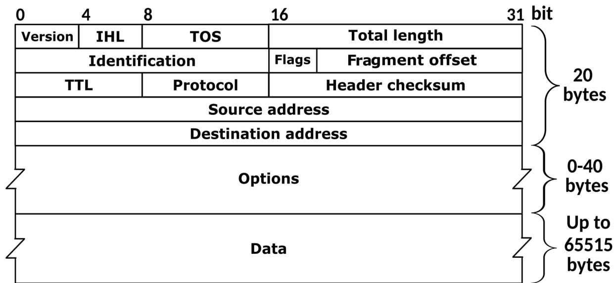
Slika 3.1. IPv4 protokol
