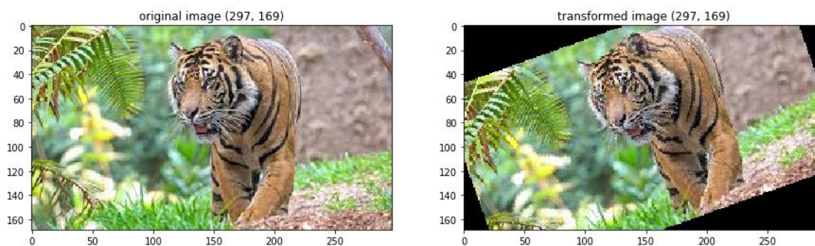
Slika 1: Rotiranje slike [14]
