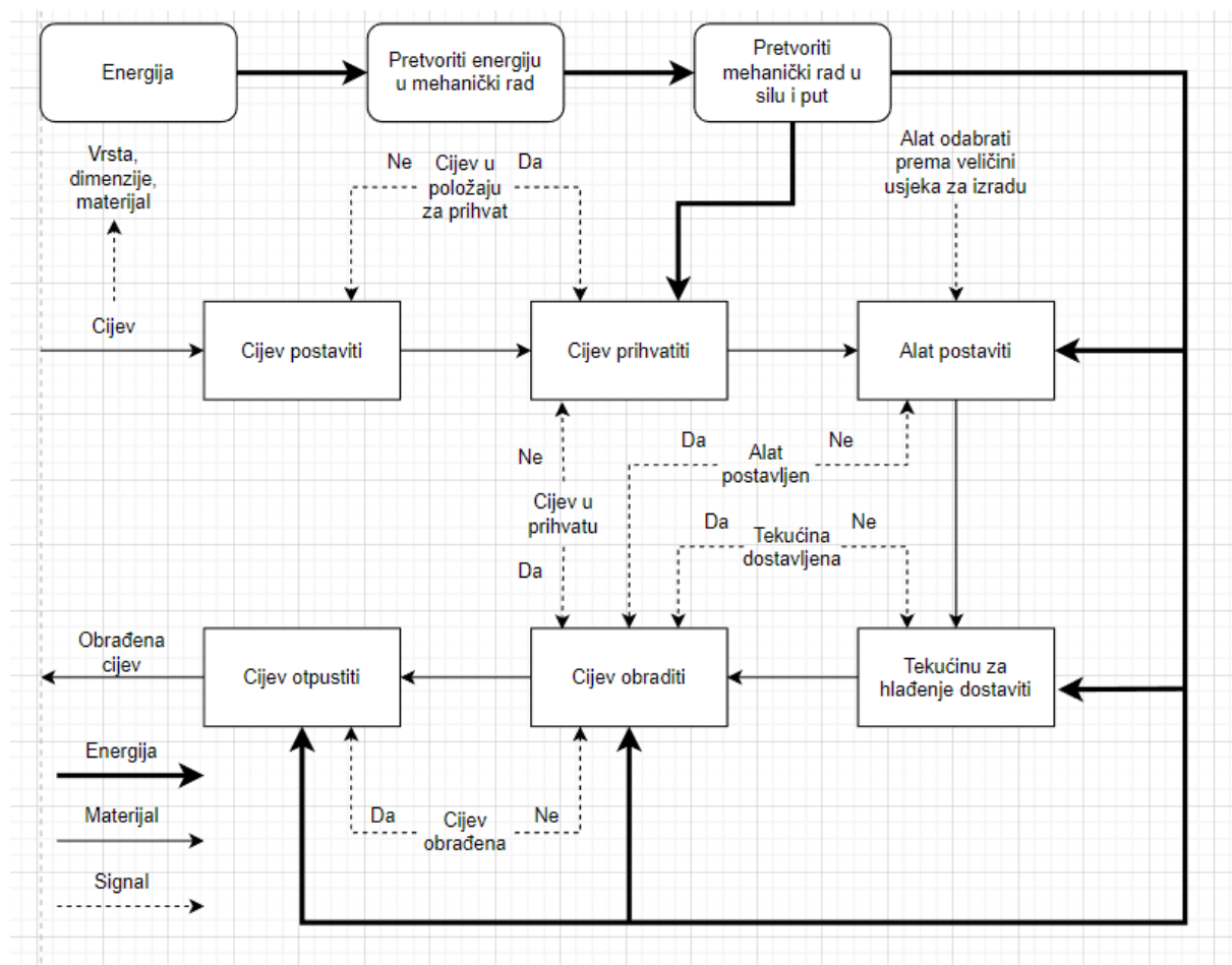
Slika 3.2 – Funkcionalna struktura [5 ]
