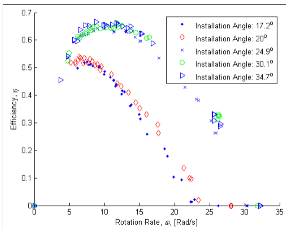
Slika 4.1.1– Odnos učinkovitosti i rotacijske brzine za različite kutove [11]
