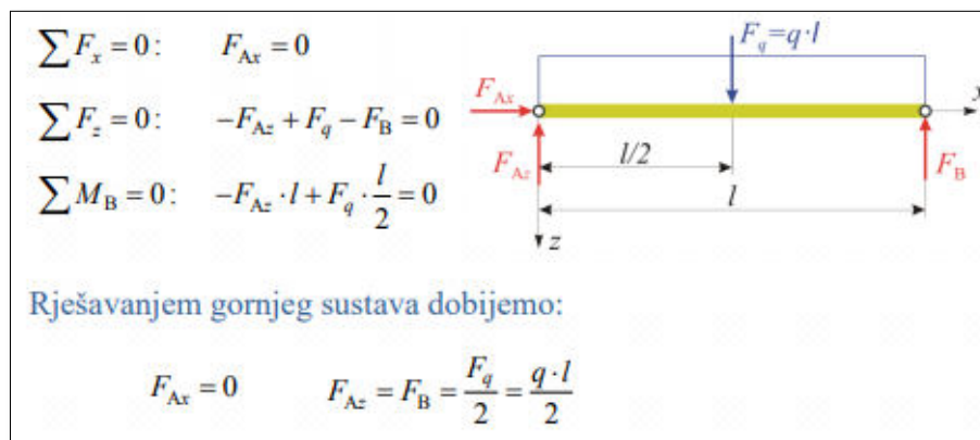
Slika 5.3- Reakcije u osloncima [13]
