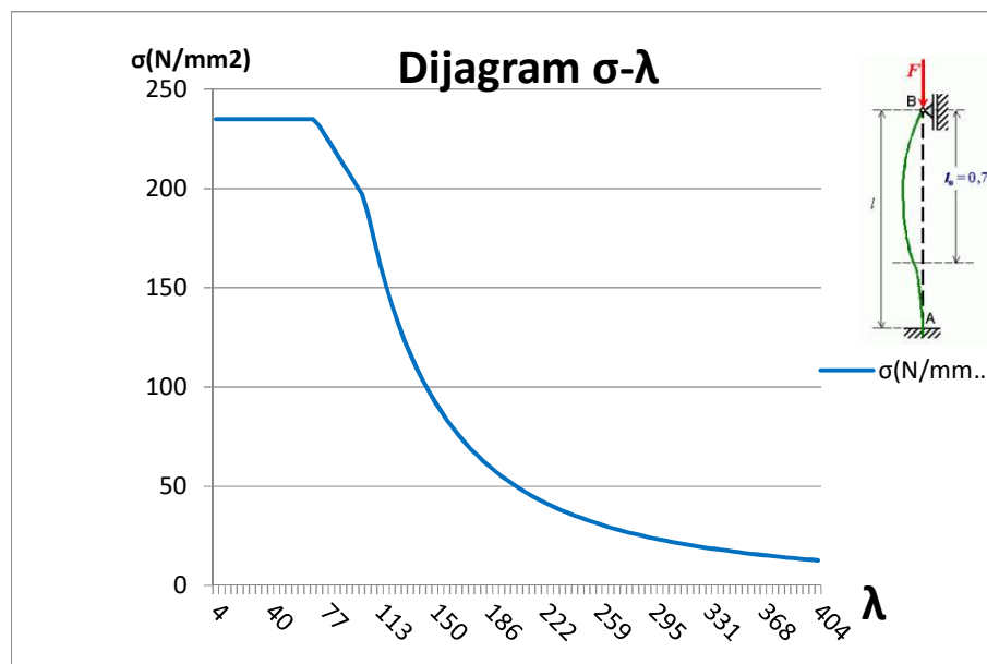
Slika 3.3 Dijagram \sigma - \lambda štapić konstrukcijskog čelika S 235 uklještjen na jednom kraju, zglobno vezan na drugom kraju
