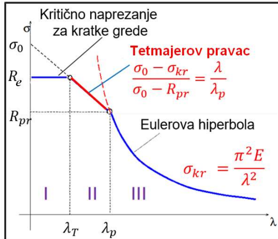
Slika 1.7 Elastično-plastično područje
