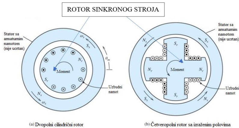
Slika12. Rotor sinkronog stroja [4]
