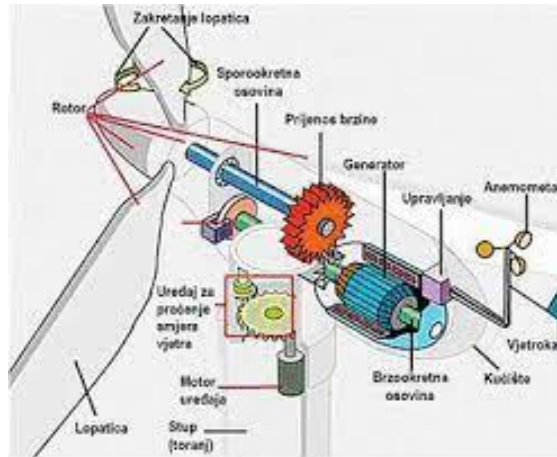
Slika 7. Kućište vjetroagregata [2]
