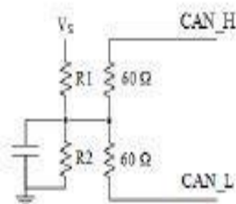
Slika 3.4. Prednaponsko razdijeljeno zaključanje
