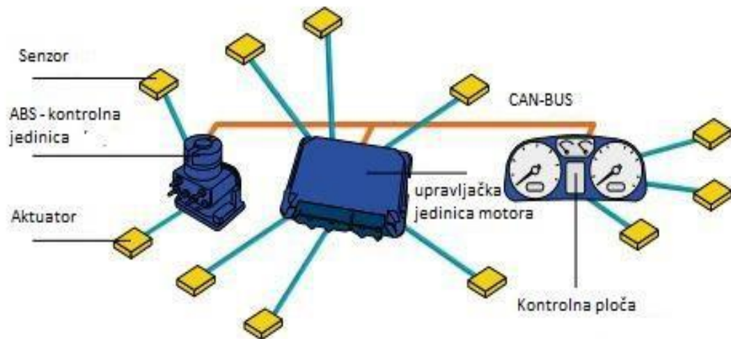
Slika 3.13. CAN mreža sklopa s 3 upravljачke jedinice [11]
