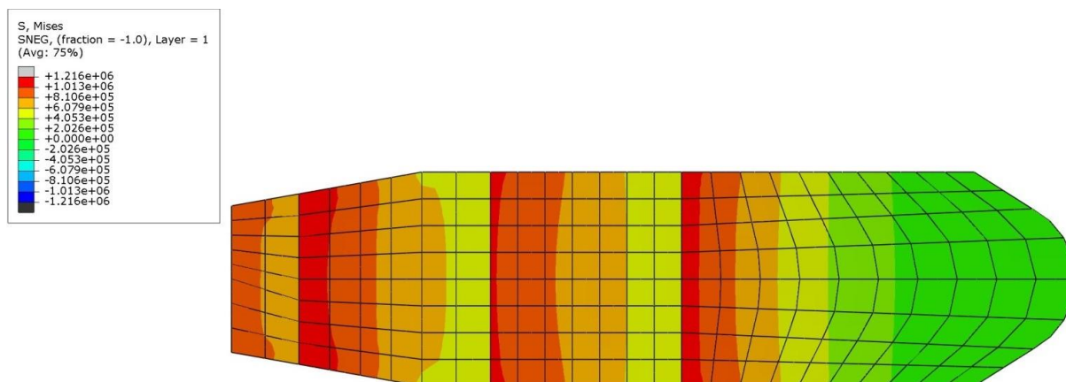
Slika 5.10 - Naprezanja u listu od staklenih vlakana
