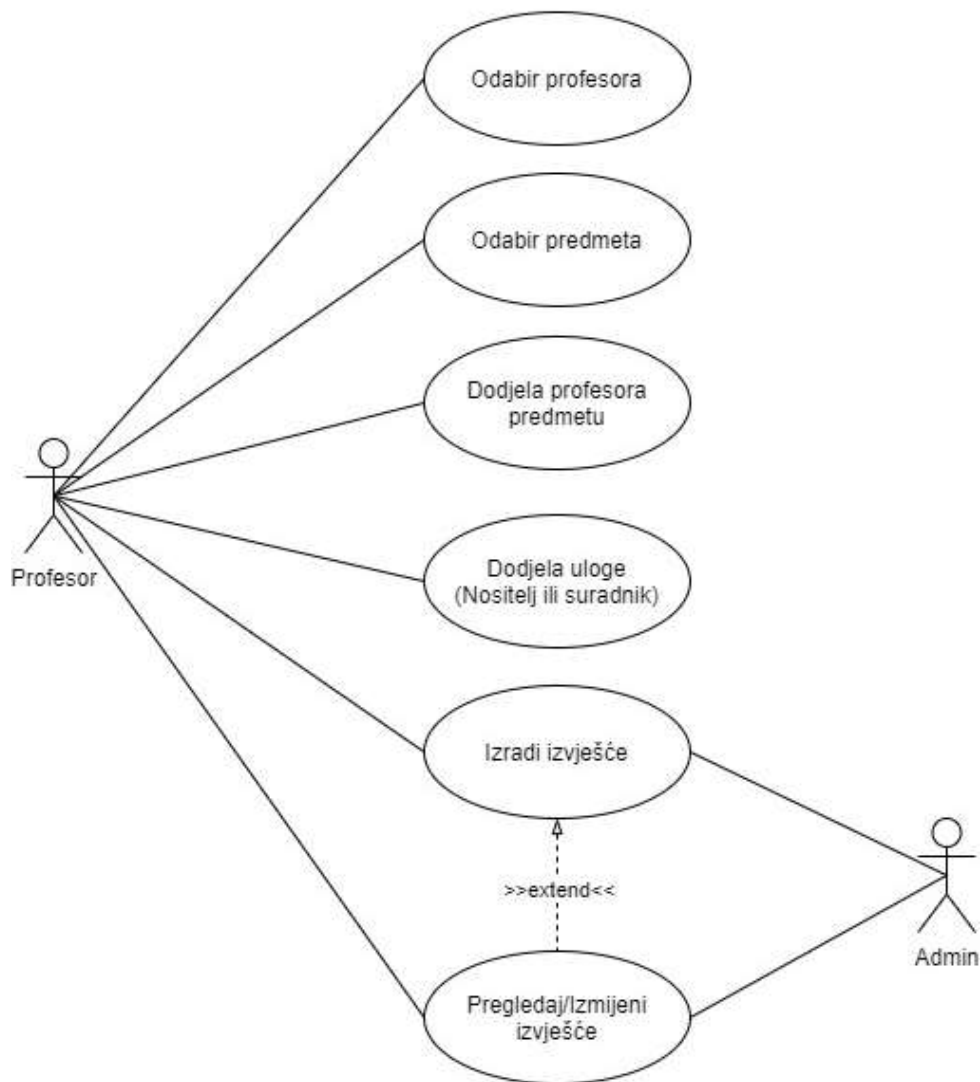
Slika 4 - dijagram slučaja uporabe za prikaz profesora i predmeta po ulogama
