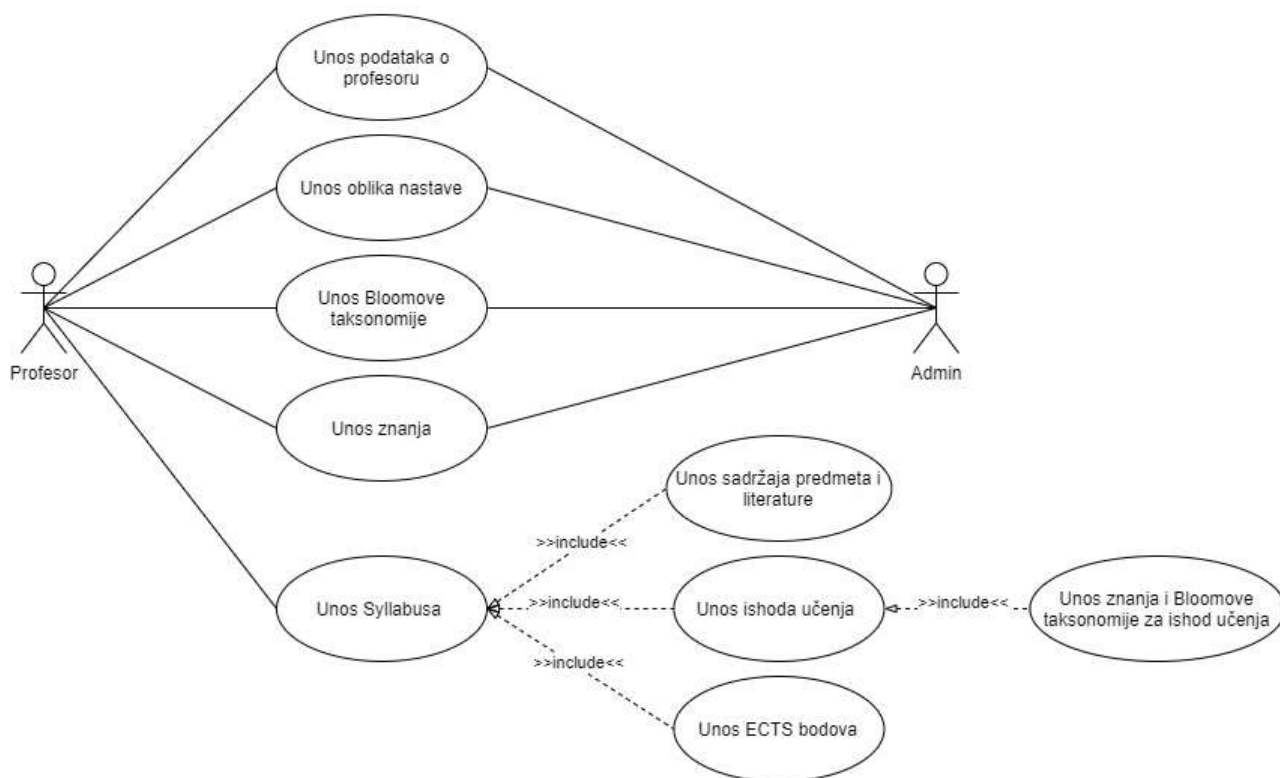
Slika 3b – dijagram slučaja uporabe za evidenciju nastavnog plana i programa
