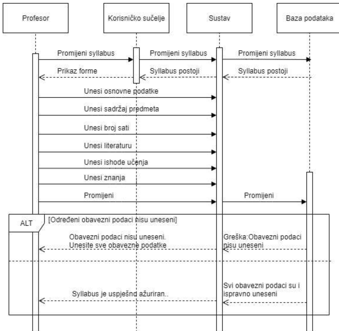
Slika 12 - dijagram slijeda za ažuriranje Syllabusa
