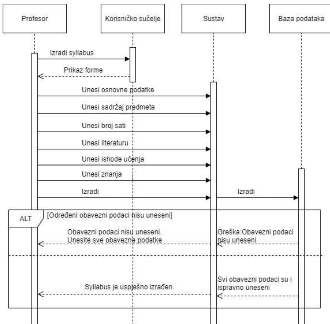
Slika 11 - dijagram slijeda za izradu Syllabusa
