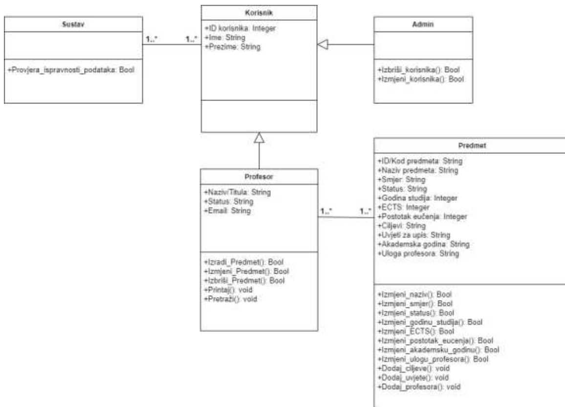
Slika 9- dijagram klasa za Profesor i Predmet
