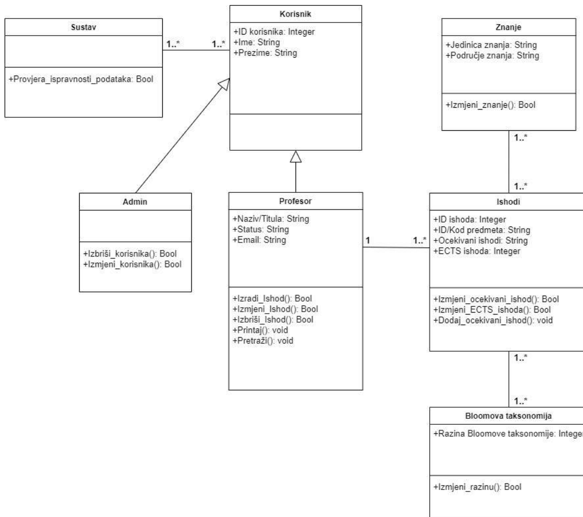
Slika 10 - dijagram klasa za ishode i znanja
