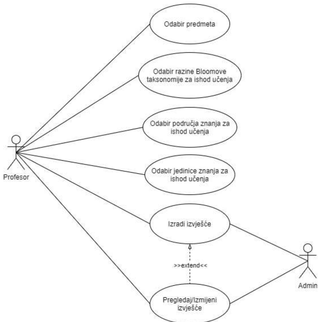
Slika 6 - dijagram slučaja uporabe za ishode učenja s dodijeljenim taksonomija
