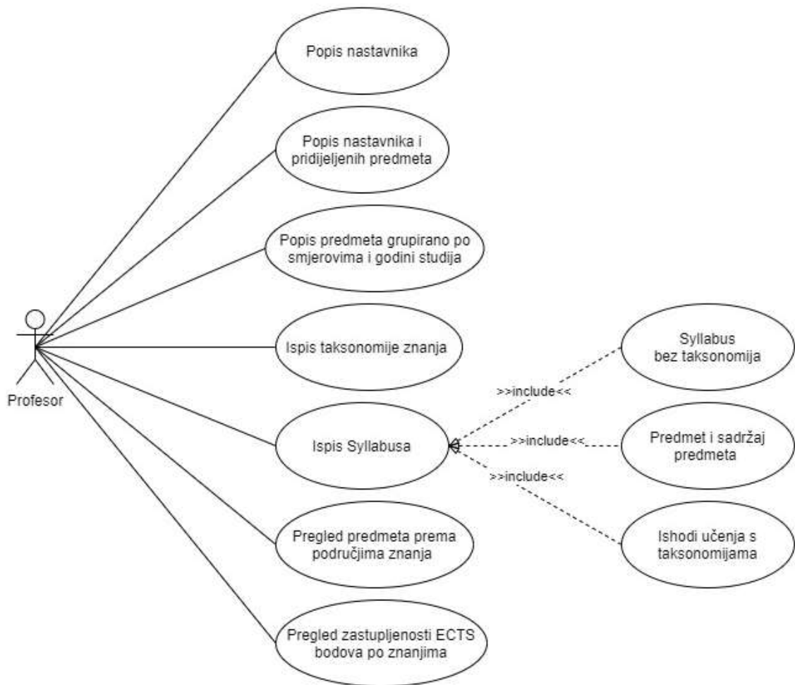
Slika 3c - dijagram slučaja uporabe za Izvješća
