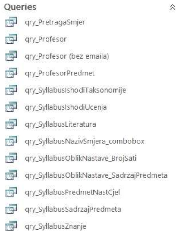
Slika 17 - popis upita
